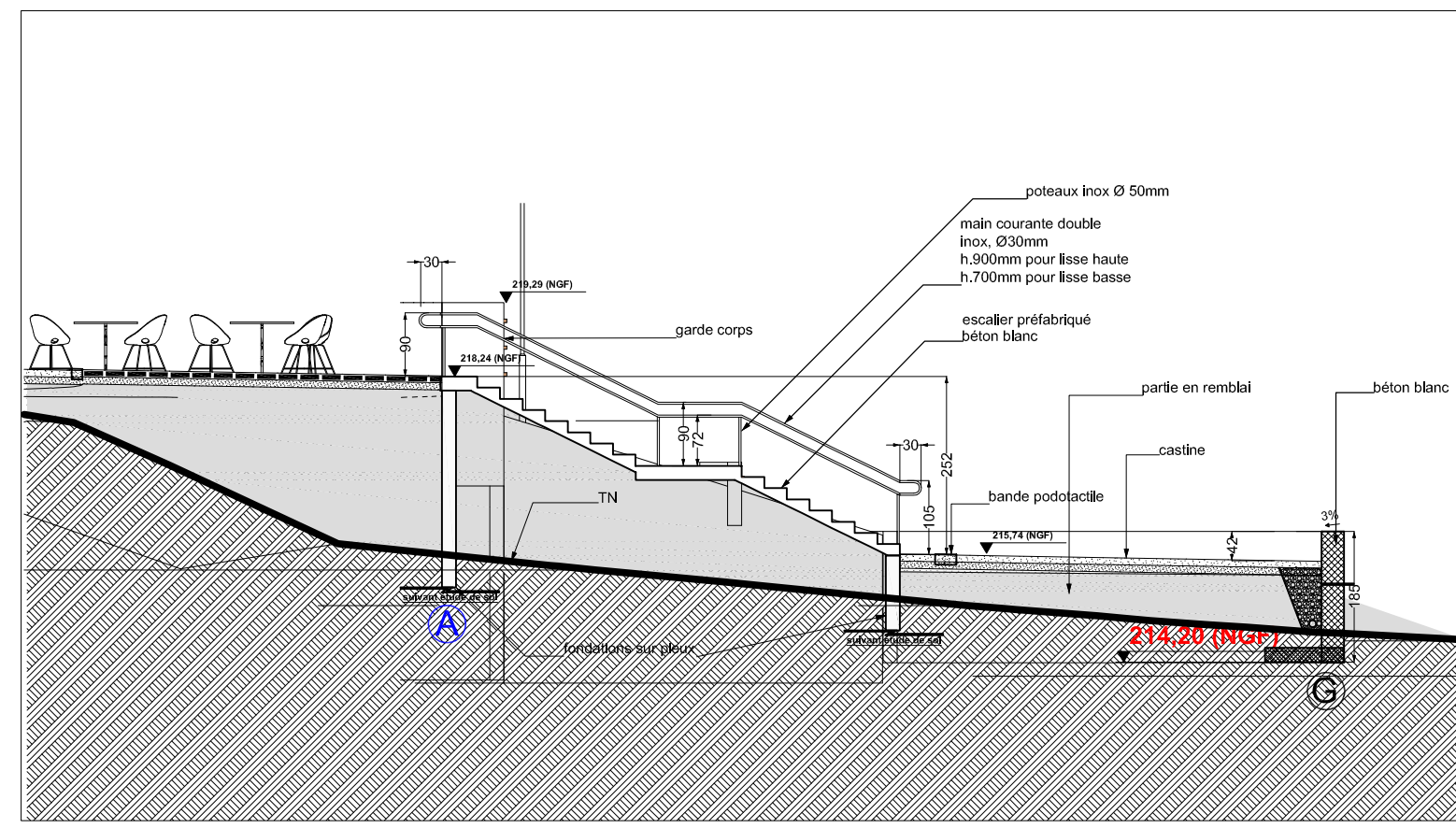
TM6 1:100 Coupe sur l'escalier entre place et parc
