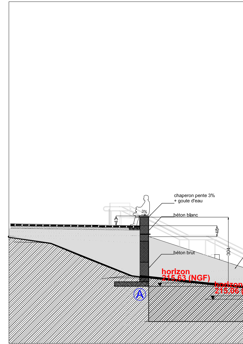
TM3 1:100 Coupe sur muret servant d'assise
