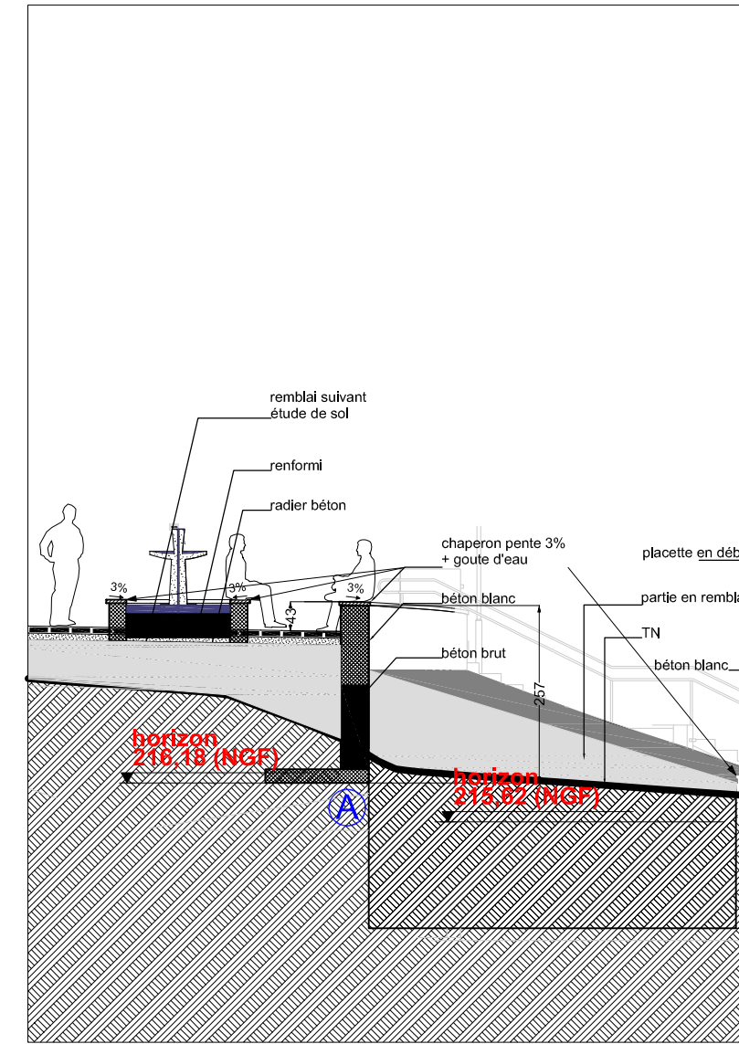
TM4 1:100 Coupe sur la fontaine à coupelle
