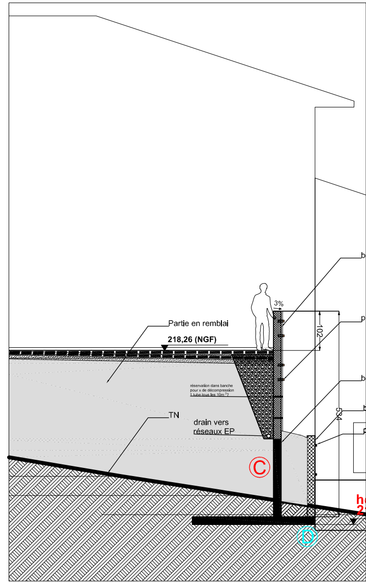
TM1 1:100 Coupe sur les murs de soutènement avec semelle unique
