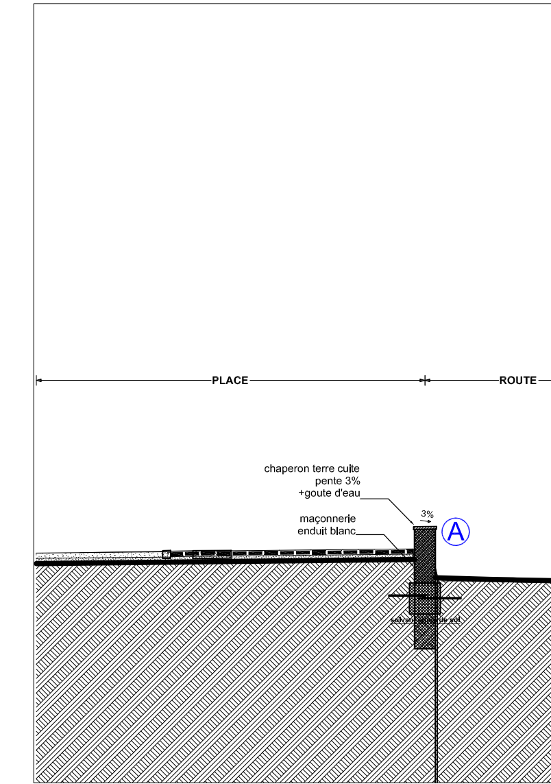
TM5 1:100 Coupe sur le mur sur semelle filante
