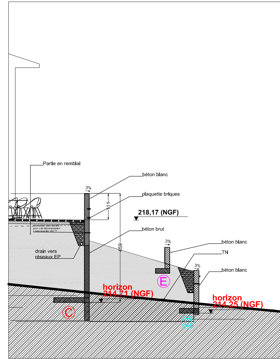
TM2 1:100 Coupe sur les murs de soutènement avec semelles indépendantes
